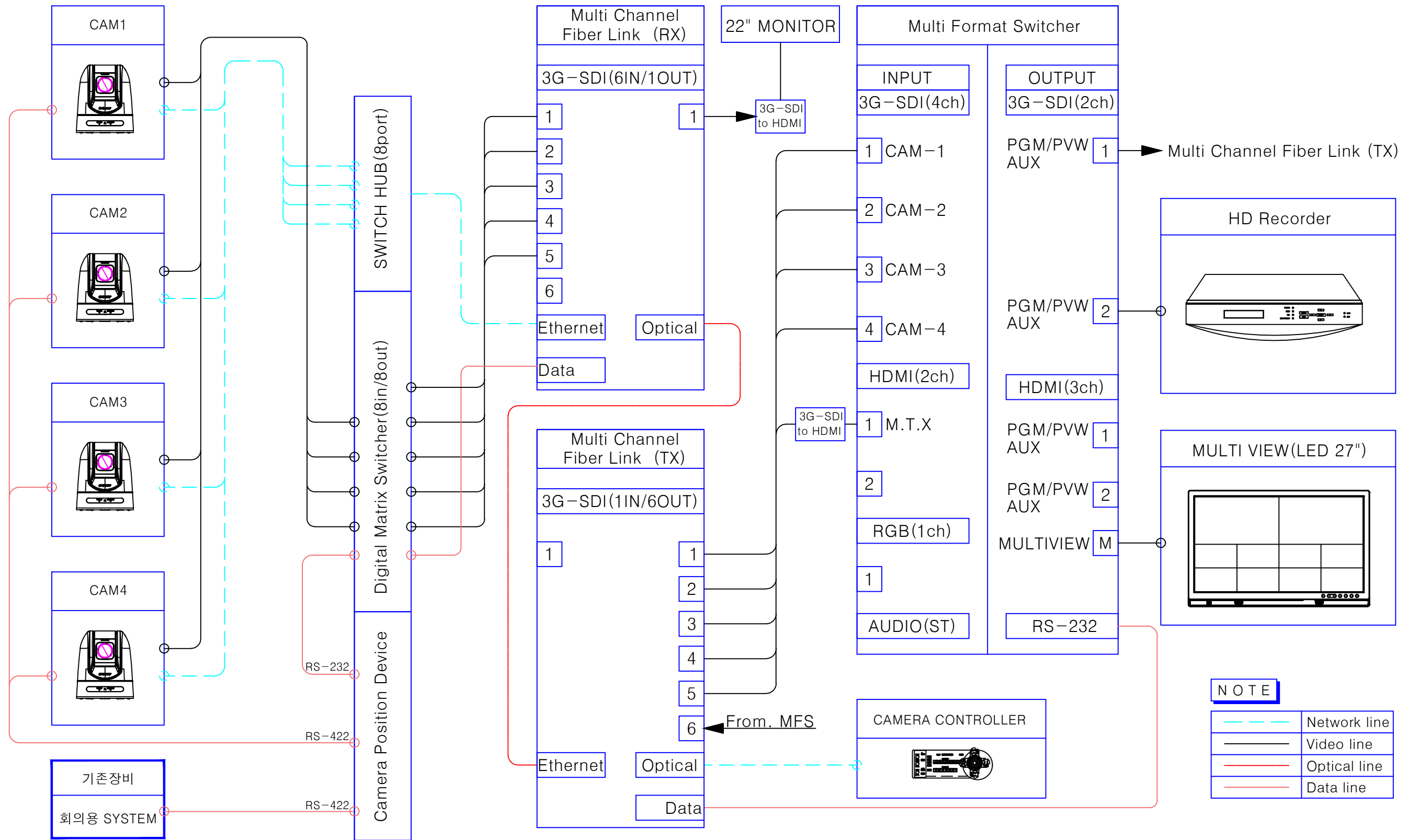
상임위원회 HD 영상시스템 BLOCK DIAGRAM SCALE: A3 1/NONE
